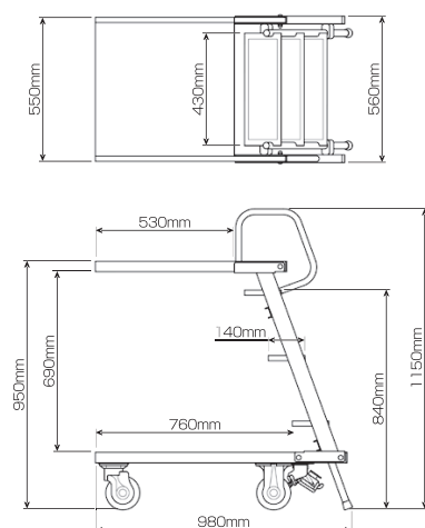
■寸法図
